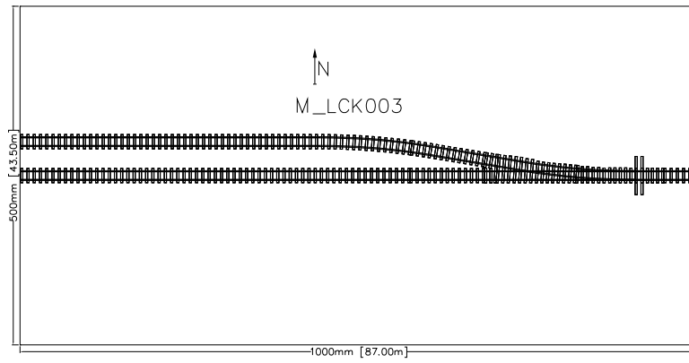
Abb. 3 Zeichnung 1:10 M_LCK003
