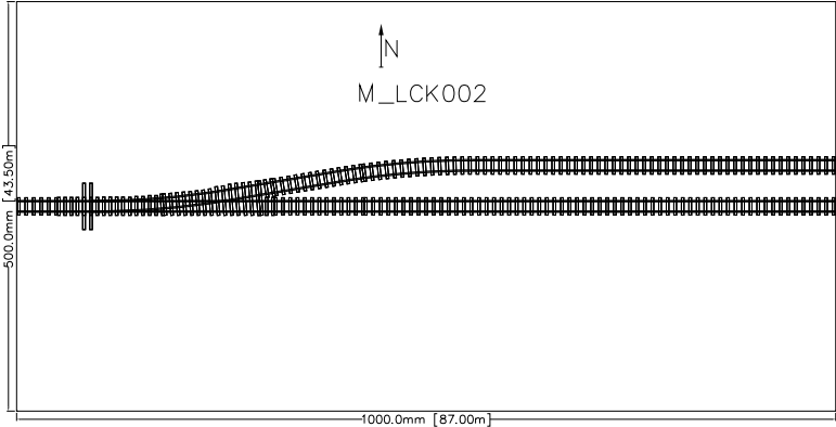
Abb. 2 Zeichnung 1:10 M_LCK002
